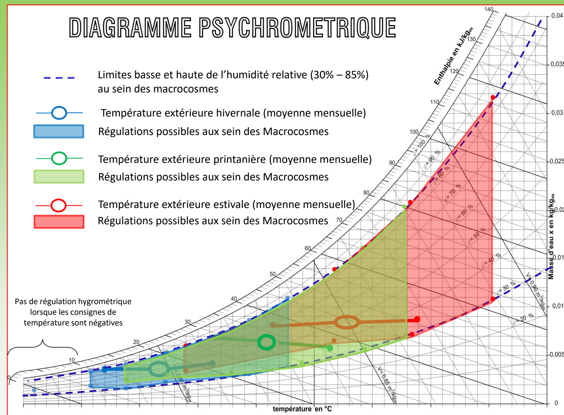
Diagramme psychrométrique sur lequel est indiqué, en fonction des saisons, les plages de fonctionnement du dispositif de conditionnement climatique Macrocosmes
