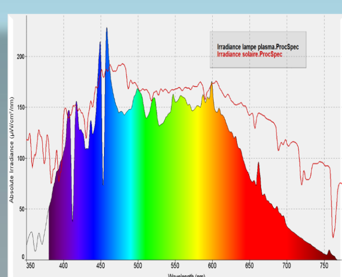
Comparaison de l'irradiance solaire (courbe rouge) et l'irradiance obtenue avec une lampe plasma dans le visible
