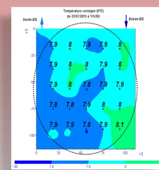
Cartographie d'homogénéité thermique de la table (test à vide)
